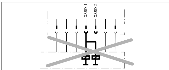
Fig. 5-7 : Ne jamais relier ensemble les sorties OSSD, la redondance disparaîtrait.
