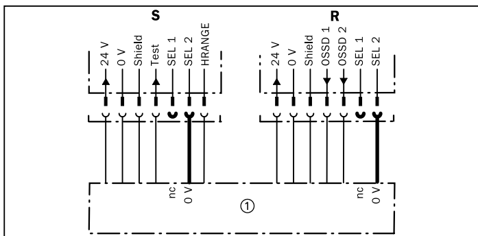
Fig. 5-9: Koplingseksempel: Tilkopling innganger kodet lys, adresse 3
