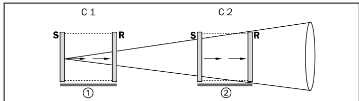
Abb. 3-4: Anordnung von Sendern und Empfängern C 2000/M 2000, Geräteversionen "Standard" und "RES/EDM" mit Strahlcodierung C 1, C 2=Strahlcodierung 1, 2 ①=System 1 ②=System 2 S=Sender R=Empfänger
