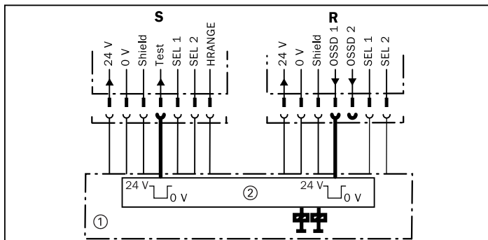
Fig. 5-8: Konfigurasjon syklisk systemtest, tilkopling testinngang og OSSD-utganger
