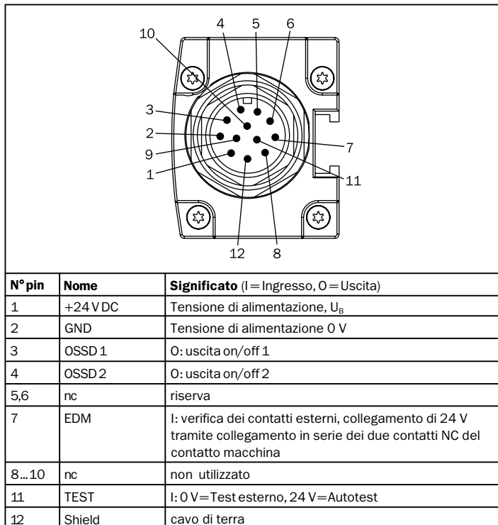
Fig. 5-3: Emittitore/ricevitore M 2000 A/P, nc = non collegato
