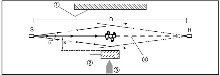
Afb. 4-1: minimum afstand tot spiegelen vlakken
