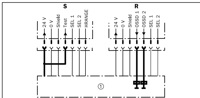
Fig. 5-6 : Raccordement des sorties OSSD pour l'autotest de l'appareil
