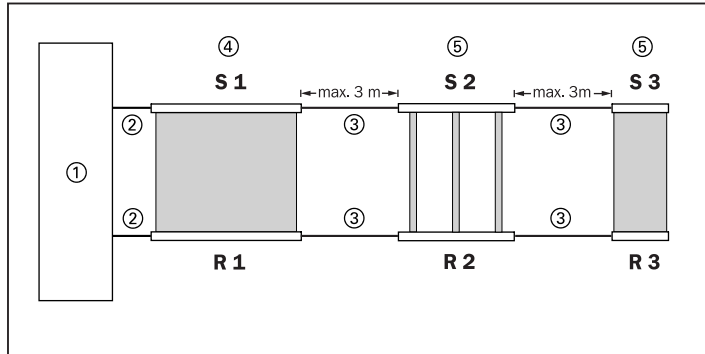
Abb. 3-5: Kaskadierung von drei Geräten C 2000/M 2000
