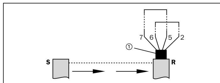
Fig. 5-13 : C 2000/M 2000 avec verrouillage redémarrage désactivée
