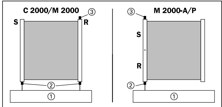
Abb. 3-3: C 2000/M 2000 mit RES/EDM und M 2000-A/P mit RES ①=Maschine ②=Systemstecker (EDM) ③=Erweiterungsstecker für RES S=Sender R=Empfänger
